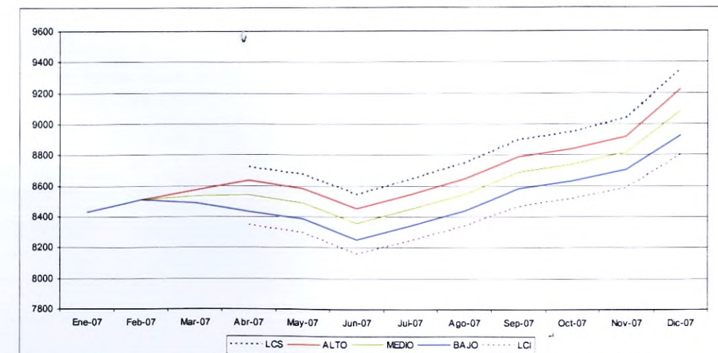
Gráfica 17 Túnel de escenarios y límites de confianza proyección mensual de potencia eléctrica en el 2007.
