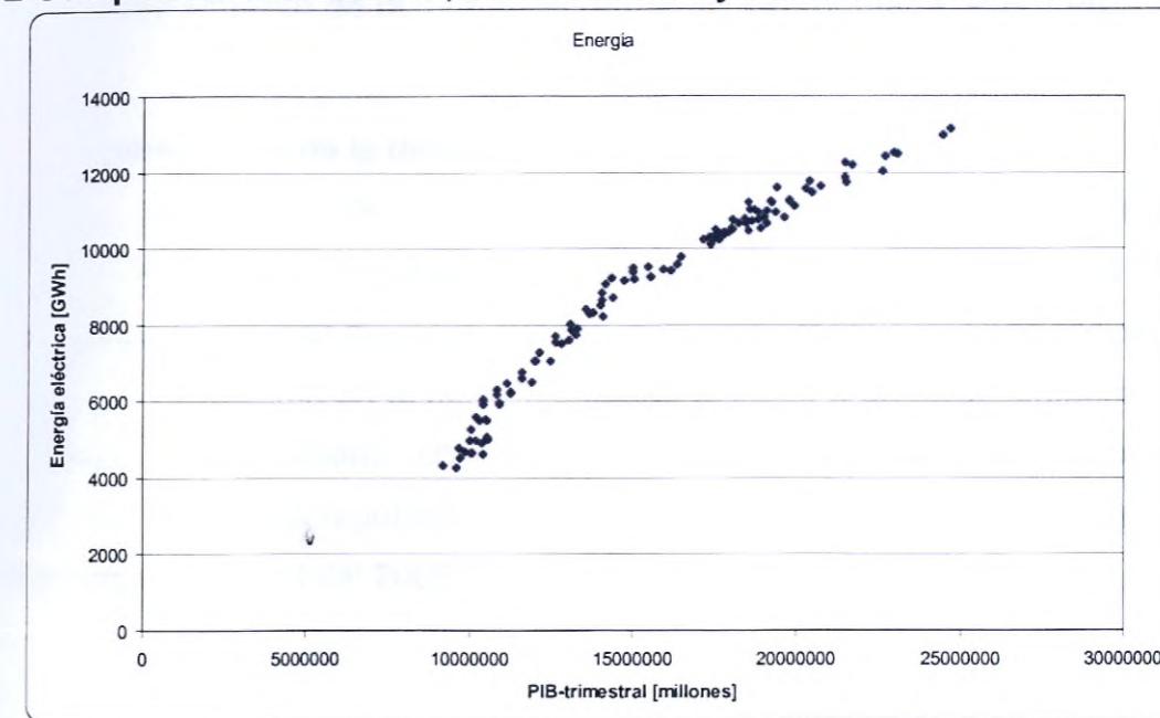
Gráfica 3 Comportamiento del PIB vs. demanda eléctrica a escala trimestral.
