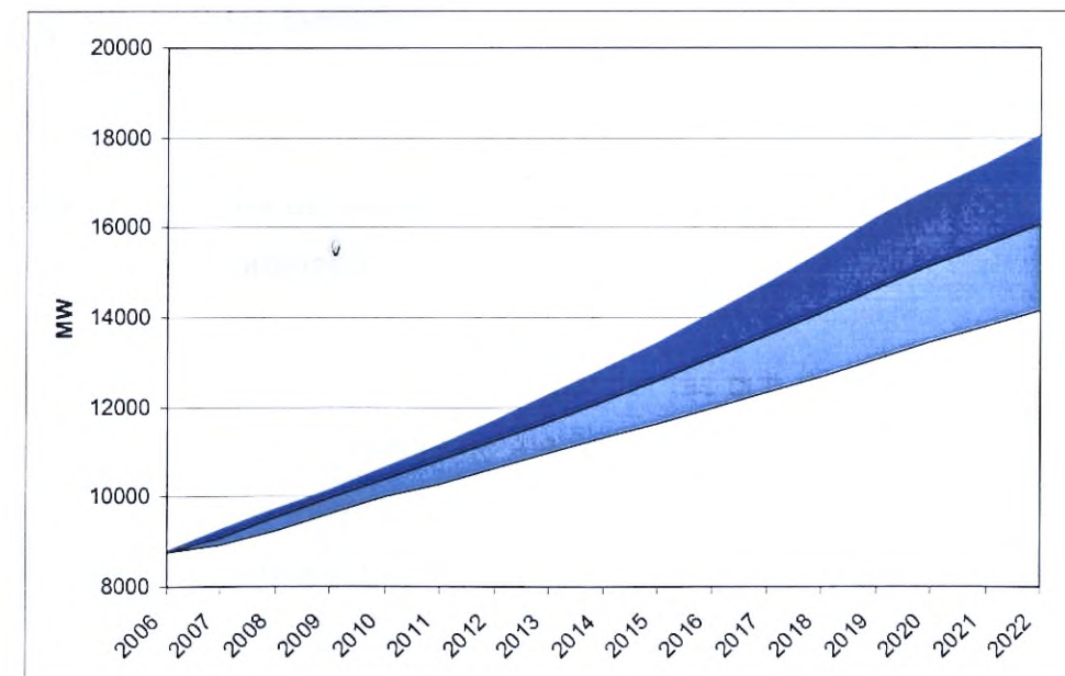
Gráfica 15. Túnel de proyección de demanda doméstica de Potencia 2007 - 2022
