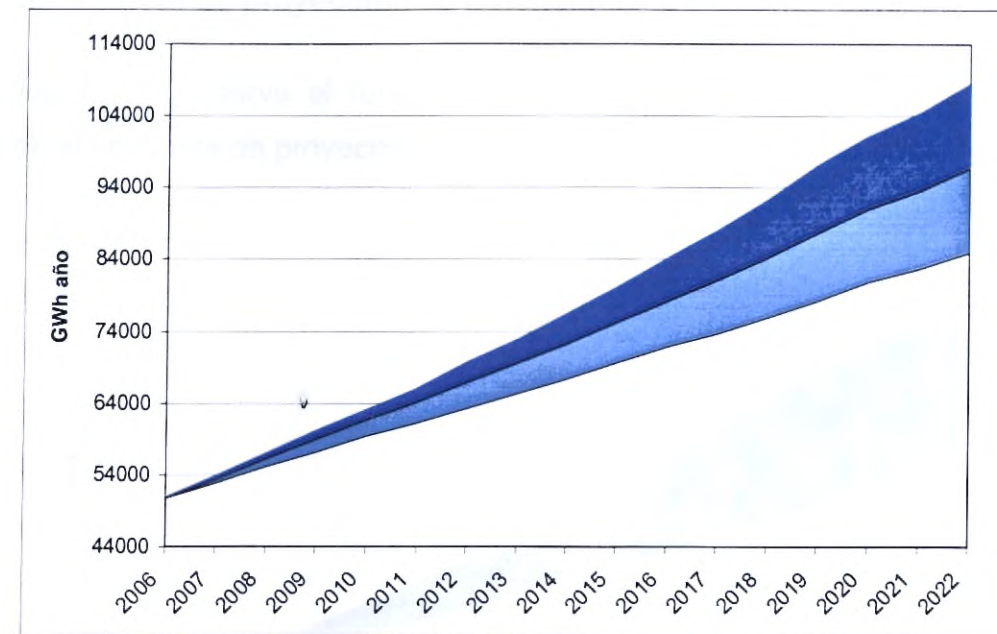
Gráfica 14. Túnel de proyección de demanda doméstica de energía eléctrica 2007-2022.
