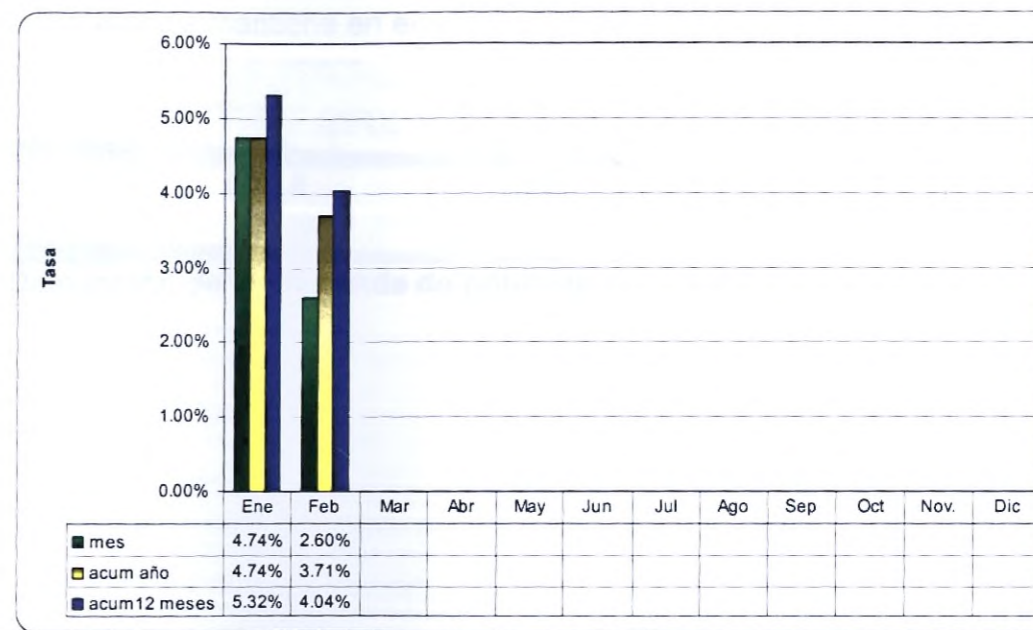
Gráfica 9 Seguimiento mensual de la demanda de energía eléctrica 2007.
