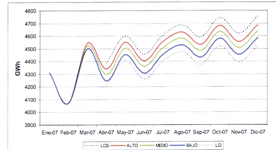
Gráfica 16 Túnel de escenarios y límites de confianza proyección mensual de energía eléctrica en el 2006.
