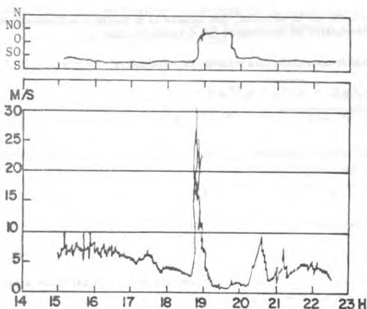
Figura 51 — Variación de la Dirección y Velocidad del Viento cuando se presenta una Turbonada
