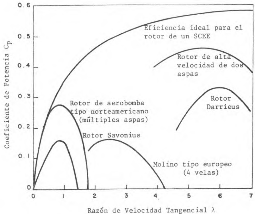
Figura 20 — Características de Potencia para Diferentes tipos de Rotores
