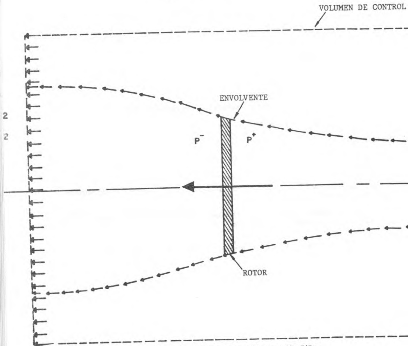
Figura 18 - Volumen de Control de una Turbina Eólica
