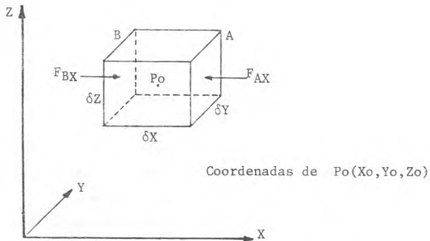
Figura 6 — Fuerza debida al gradiente de presión (descripción)
