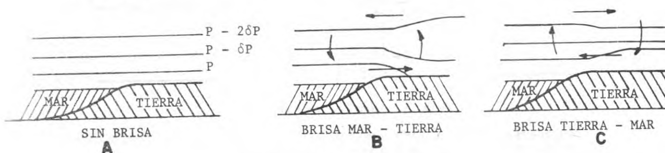
Figura 14 — Brisas de Tierra y de Mar
