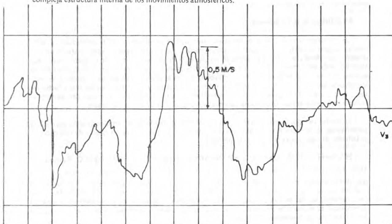
Figura 46 — Registros Típicos de la Variación Temporal de la Componente Horizontal de la Velocidad del Viento
