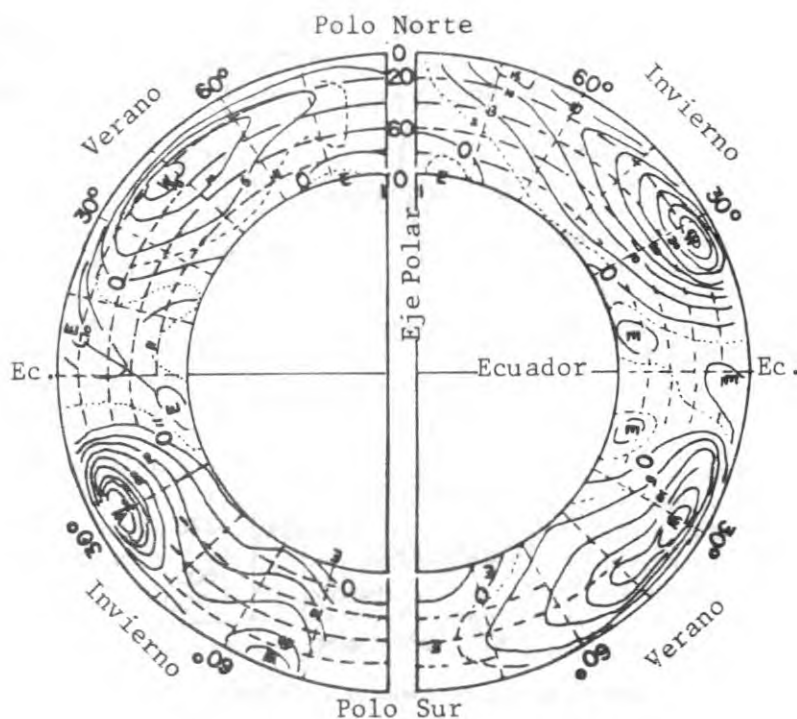
Figura 2 — Componente Zonal del Viento
