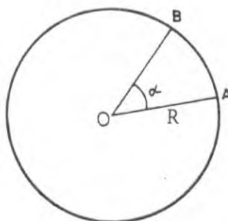
Figura 11 — Fuerza de Coriolis (descripción)
