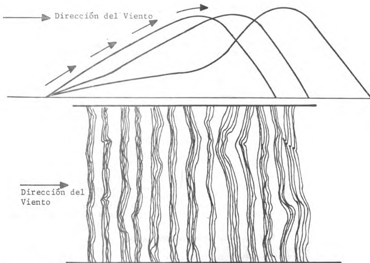
Figura 39 — Formación de Dunas
