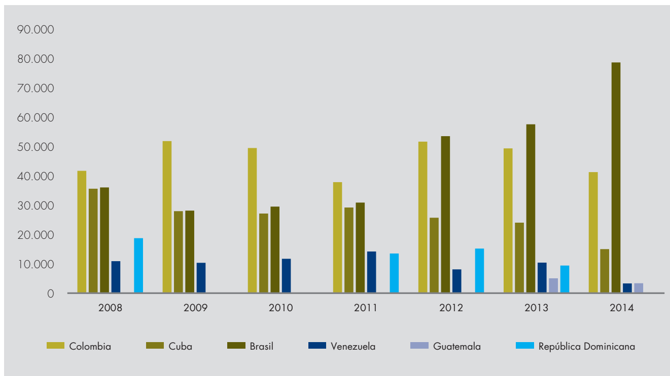
FIGURA 24. PRODUCCIÓN DE NÍQUEL EN LATINOAMÉRICA (TONELADAS/AÑO)
