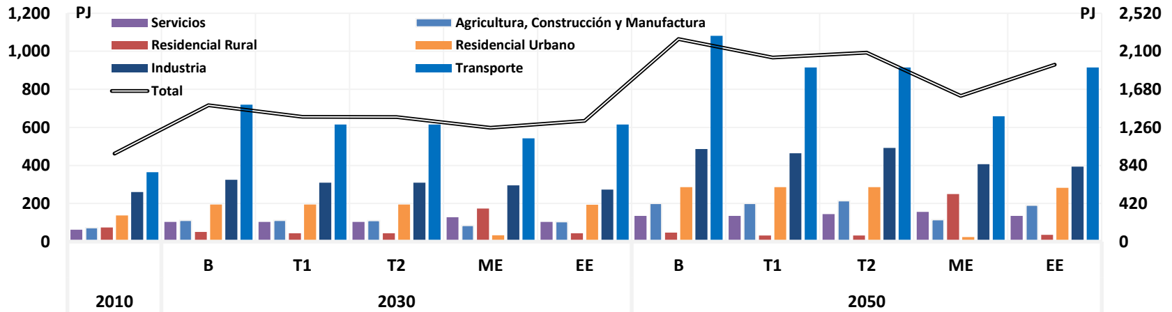
Gráfica 5-7. Demanda energética en los sectores de consumo final – Escenarios propuestos (PJ)
