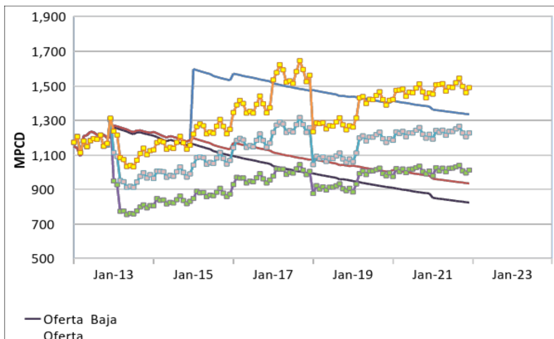
Gráfica 4-5 Balance de Gas Total
