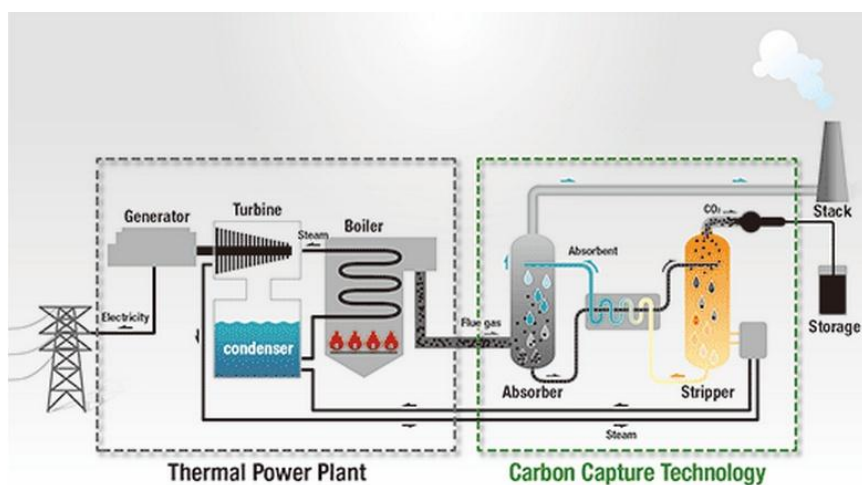
Gráfica 2-7 Captura de Carbono en una Central Térmica con Caldera
