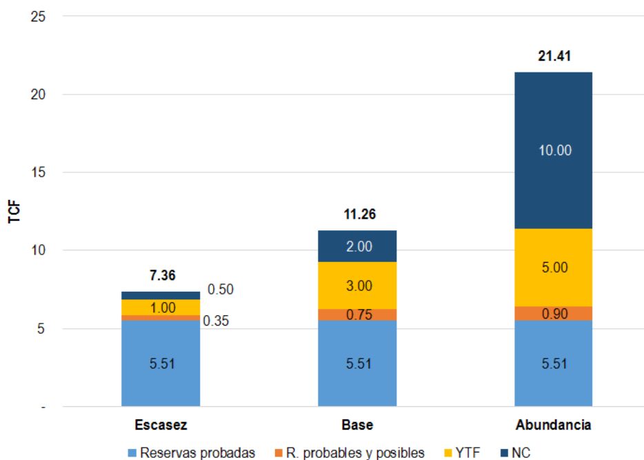
Gráfica 4-4. Escenarios de incorporación de reservas de Gas Natural
