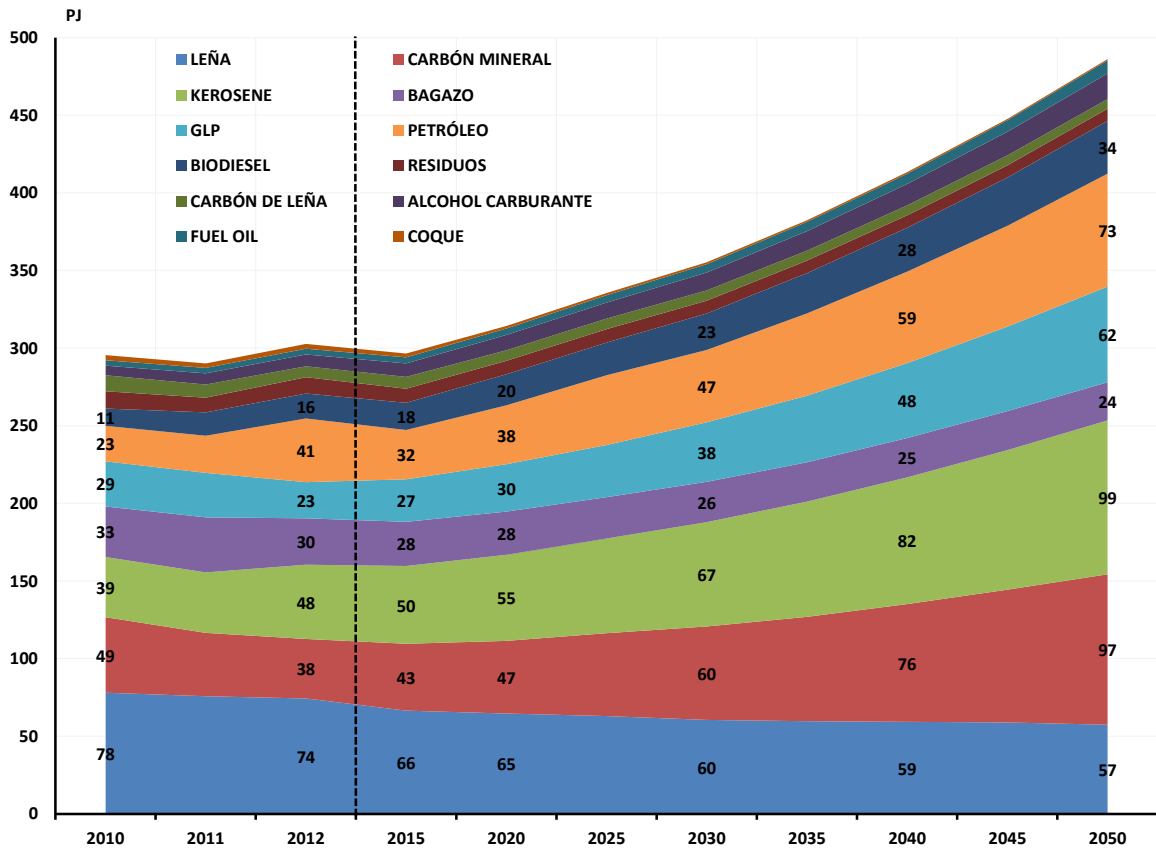
Gráfica 5-2. Evolución de la demanda por otros energéticos – Escenario Base (PJ)
