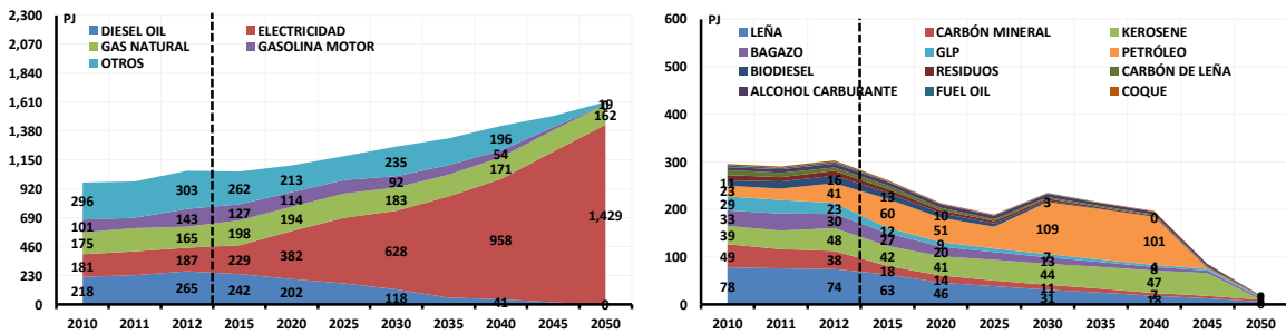
Gráfica 5-11. Evolución demanda por energéticos, Escenario ME (PJ)
