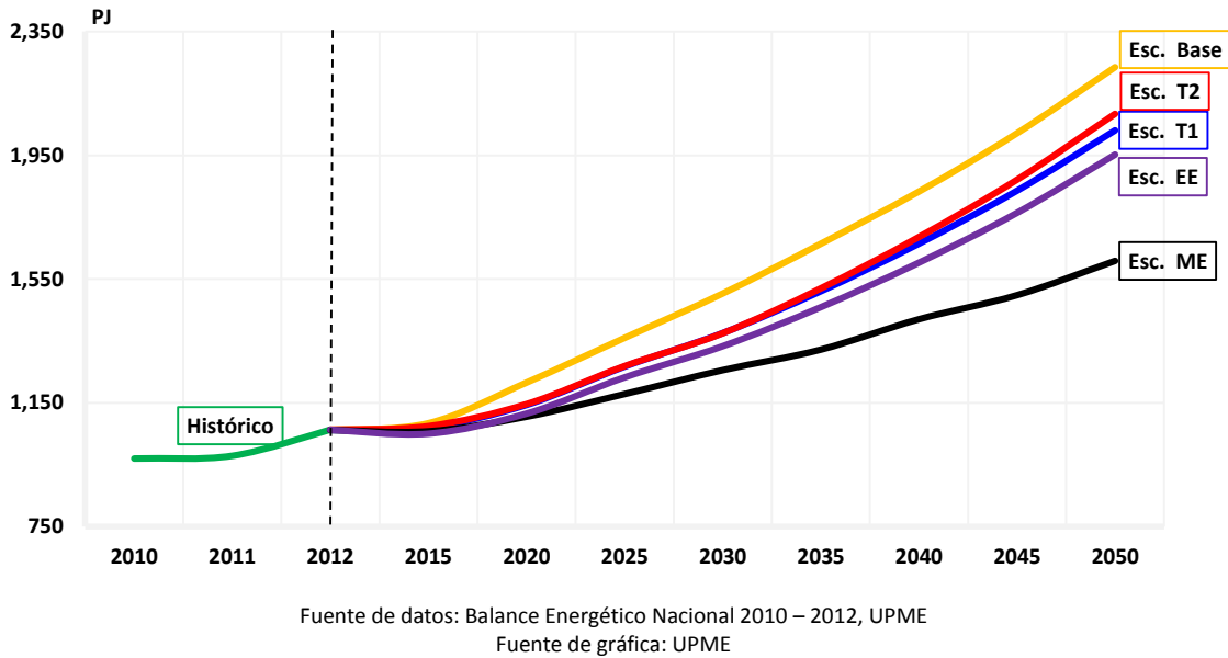
Gráfica 5-13. Evolución demanda por energéticos sectores de consumo final (PJ)
