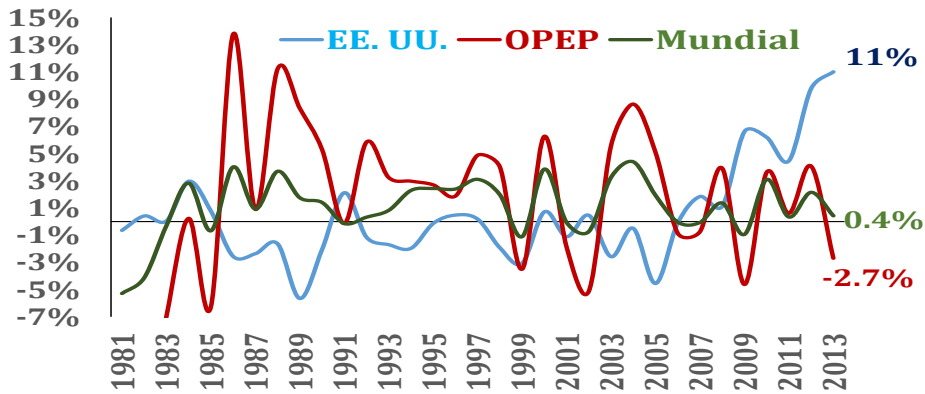
Gráfica 3-28 Crecimiento Anual de la Producción Mundial de Petróleo y Derivados
