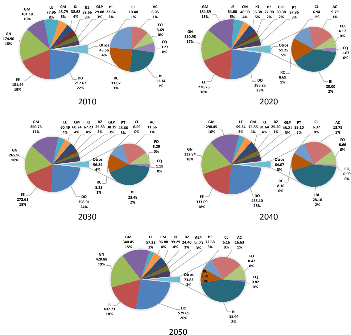
Gráfica 5-4. Evolución de la composición de la matriz energética, Consumo Final. – Escenario Base (PJ)
