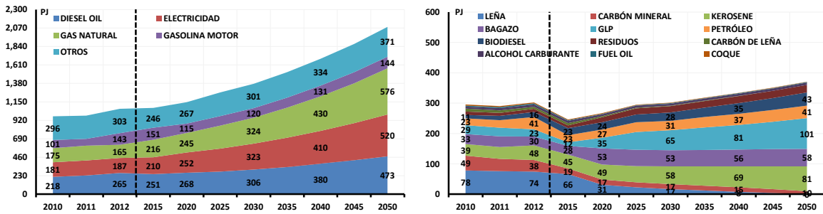
Gráfica 5-10. Evolución demanda por energéticos, Escenario T2 (PJ)
