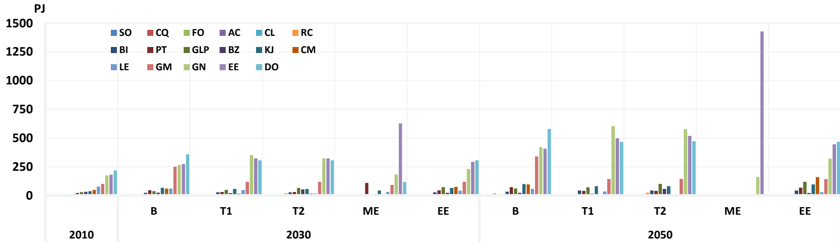
Gráfica 5-6. Demanda por energético en los sectores de consumo final – Escenarios propuestos (PJ)
