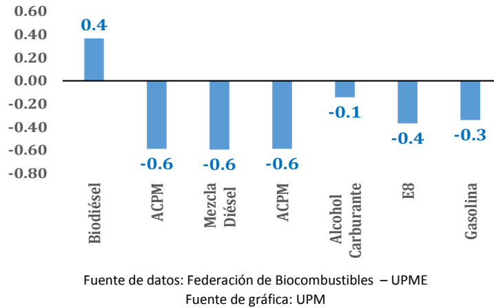
Gráfica 3-57 Variación Combustibles Biomasa Vs Variación Dólar (COP / USD)
