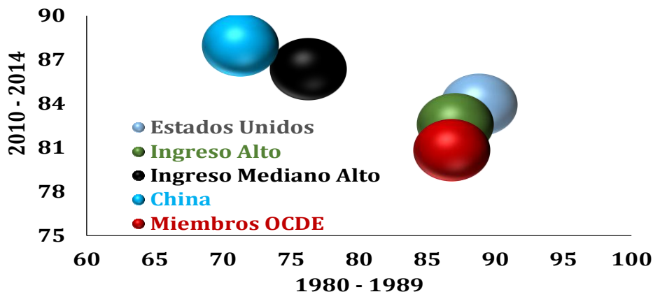
Gráfica 3-30 Porcentaje de Consumo Energía proveniente de Combustibles Fósiles
