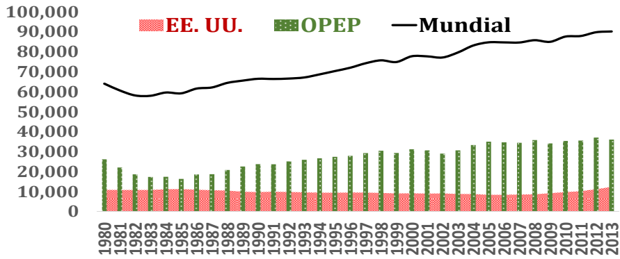
Gráfica 3-27 Composición Actual de la Producción Mundial de Petróleo
