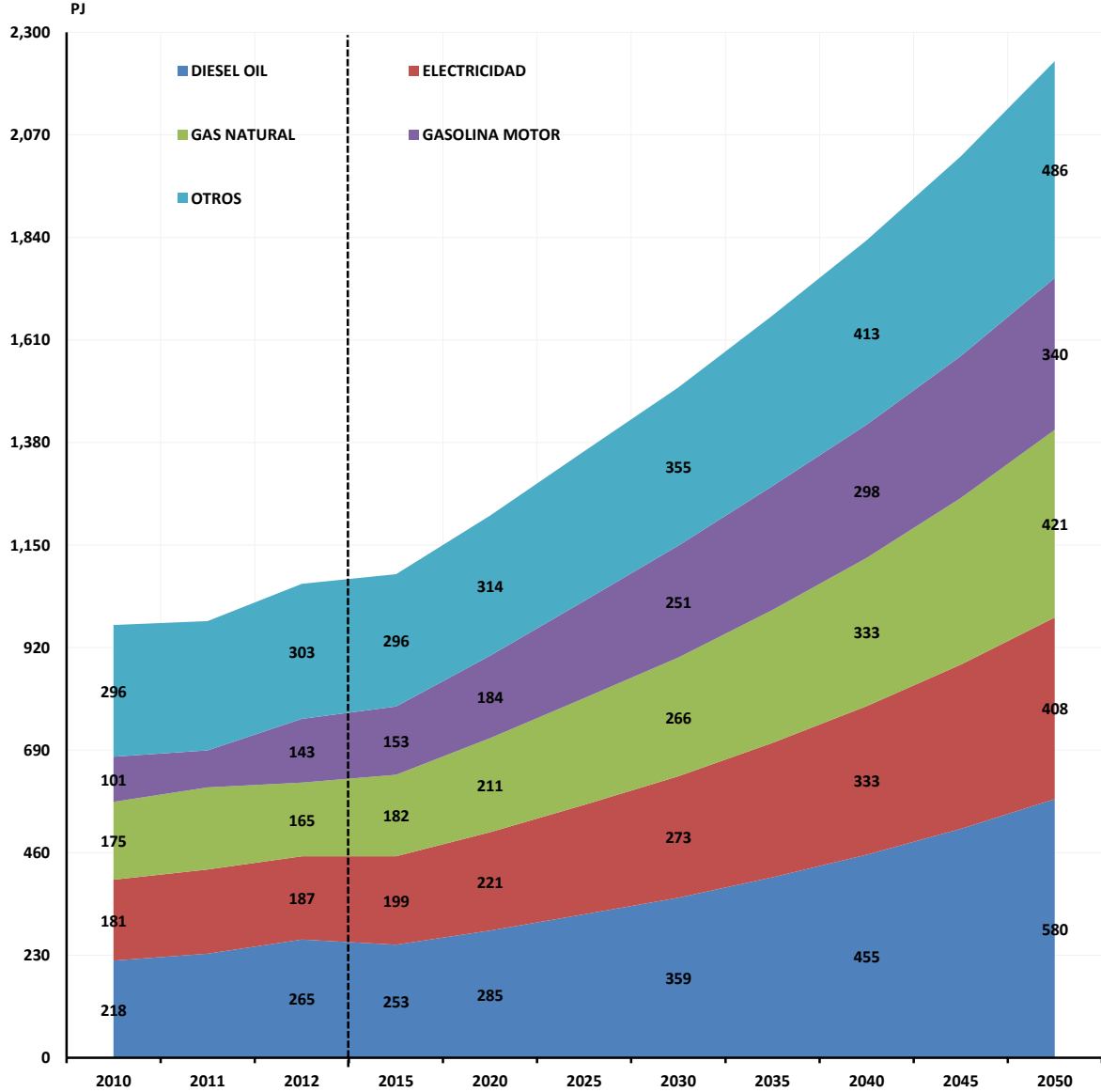
Gráfica 5-1. Evolución de la demanda por energéticos principales – Escenario Base (PJ)
