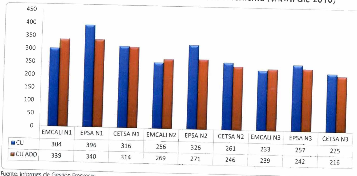
Gráfico 2-43. CU por nivel de Tensión en ADD Occidente ($/kWh dic 2010)
