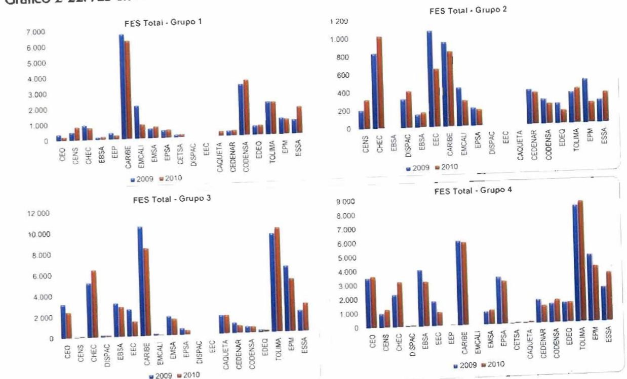
Gráfico 2-22. FES en Número de Interrupciones por Grupo de Calidad y por Empresa 2009 y 2010
