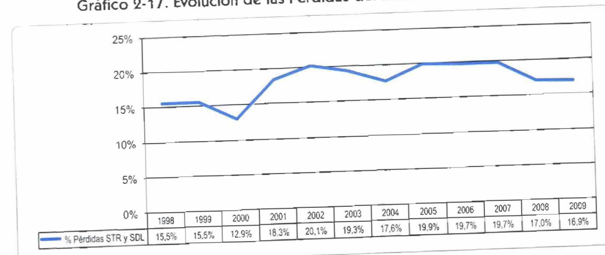
Gráfico 2-17. Evolución de las Pérdidas del Sistema de Distribución
