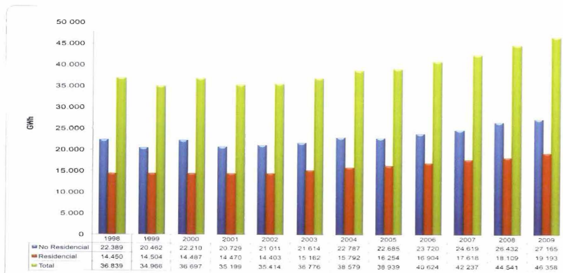
Gráfico 1-6. Evolución del Consumo de Energía Eléctrica Total Nacional 1998-2009
