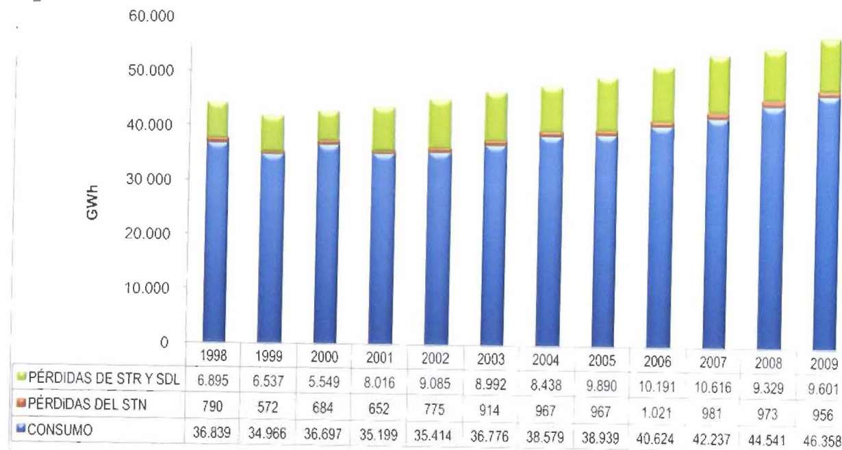
Gráfico 1-16 Evolución del Consumo y las Pérdidas del Sistema 1998-2009
