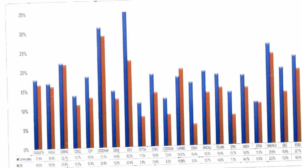
Gráfico 2-19. Pérdidas Comerciales y del OR por Empresas a Diciembre de 2010
