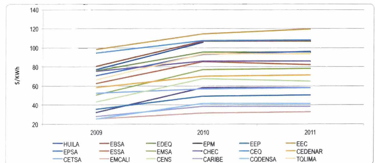
Gráfico 2-50 Cargos Máximos de Distribución Nivel de Tensión 2 (Cifras en Pesos de Diciembre de 2007)
