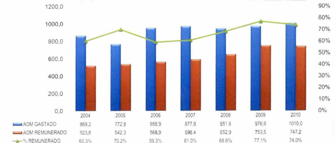
Gráfico 12. Costos AOM Remunerados y Gastados por las Empresas 2004-2010 (Cifras en Miles de Millones de Pesos Constantes de Diciembre de 2010)
