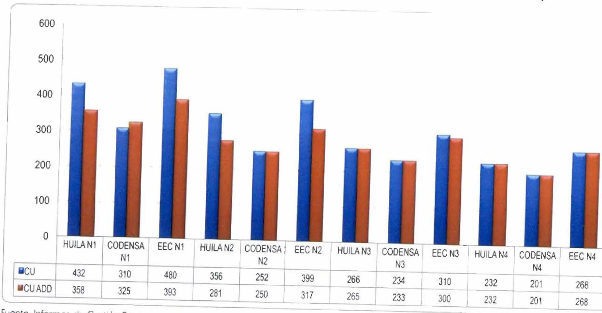
Gráfico 2-42. CU por Nivel de Tensión ADD Oriente ($/kWh dic 2010)
