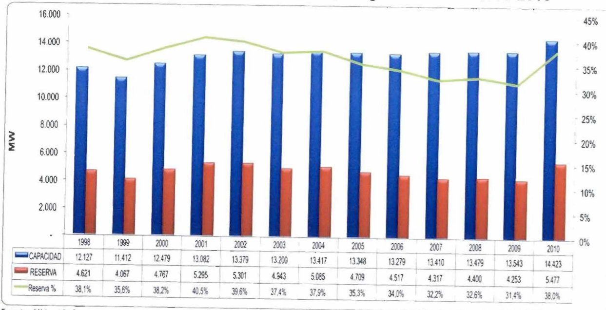
Gráfico 1-19. Capacidad Efectiva Neta y Margen de Reserva 1998-2010
