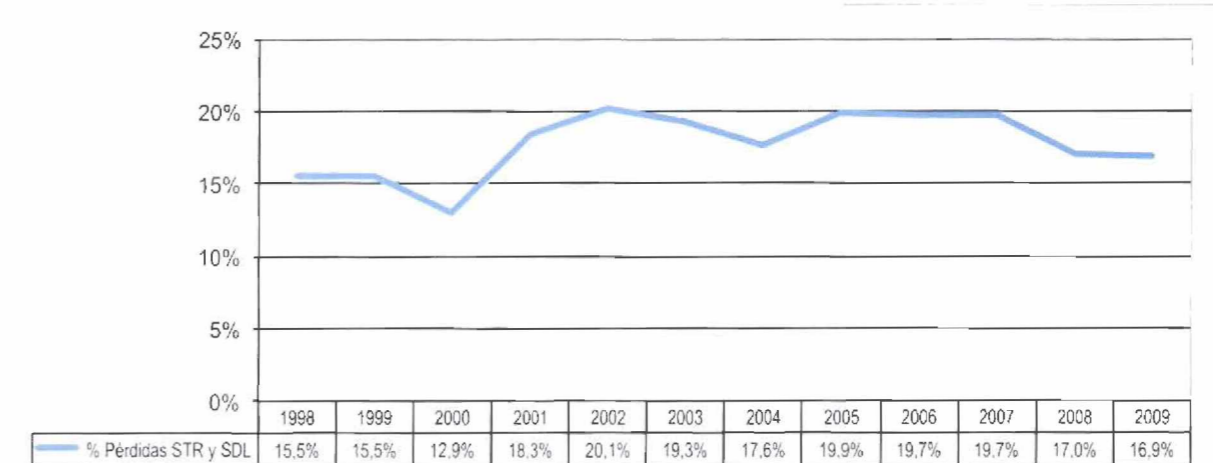
Gráfico 4. Evolución de las Pérdidas de Distribución 1998-2009
