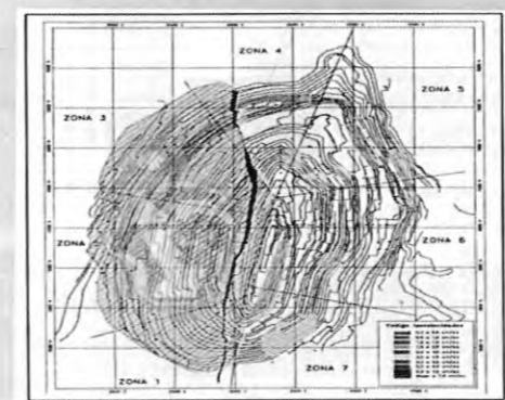
ISODESPLAZAMIENTOS MES DE MARZO 2001 DE PARED OESTE.
