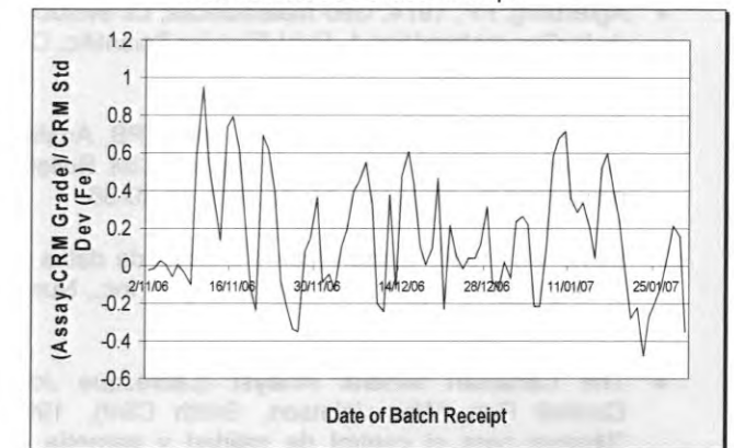
Figure 24. Promedio móvil de resultados de Fe normalizados versus Tiempo
