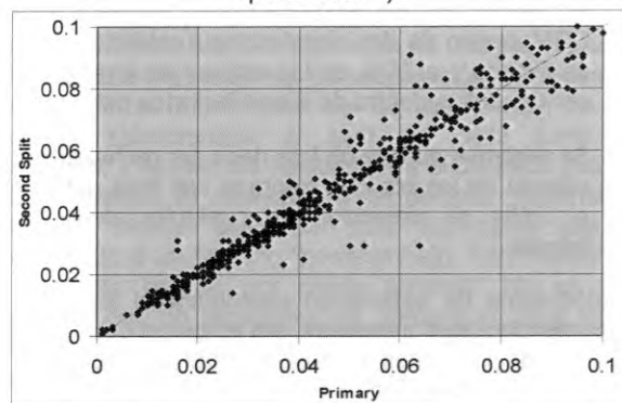
Figure 15. Gráfico de dispersión de pares de muestras (710 duplicados de rechazos de muestras analizadas para fósforo)
