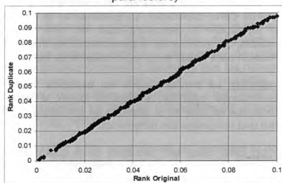
Figure 16. Gráficos Quantil-Quantil de muestras pareadas (710 duplicados de rechazos de muestras analizadas para fósforo)
