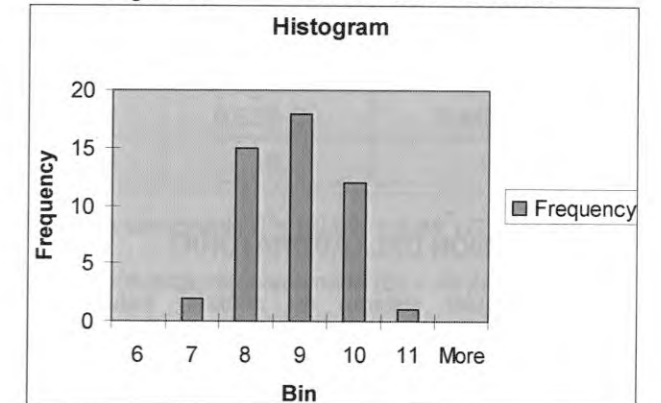
Figure 19. Distribución de los datos
