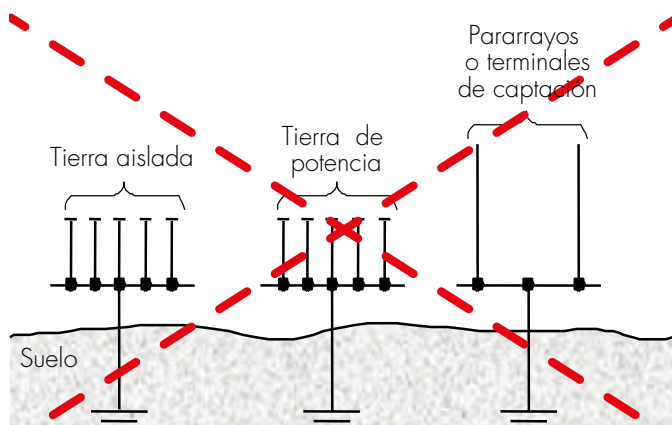
Figura 15.3. Una sola puesta a tierra para todas las necesidades
