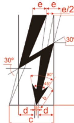
Figura 6.1. Símbolo de riesgo eléctrico
