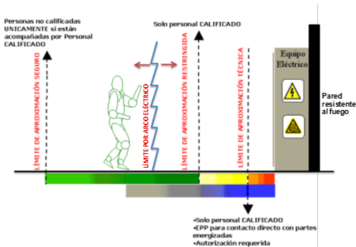
Figura 13.4. Límites de aproximación
