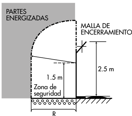
Figura 23.1. Distancias de seguridad para prevenir contactos directos en subestaciones exteriores
