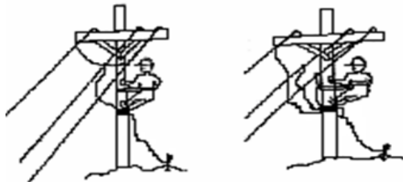
Figura 15.6. Montajes típicos de puestas a tierra temporales
